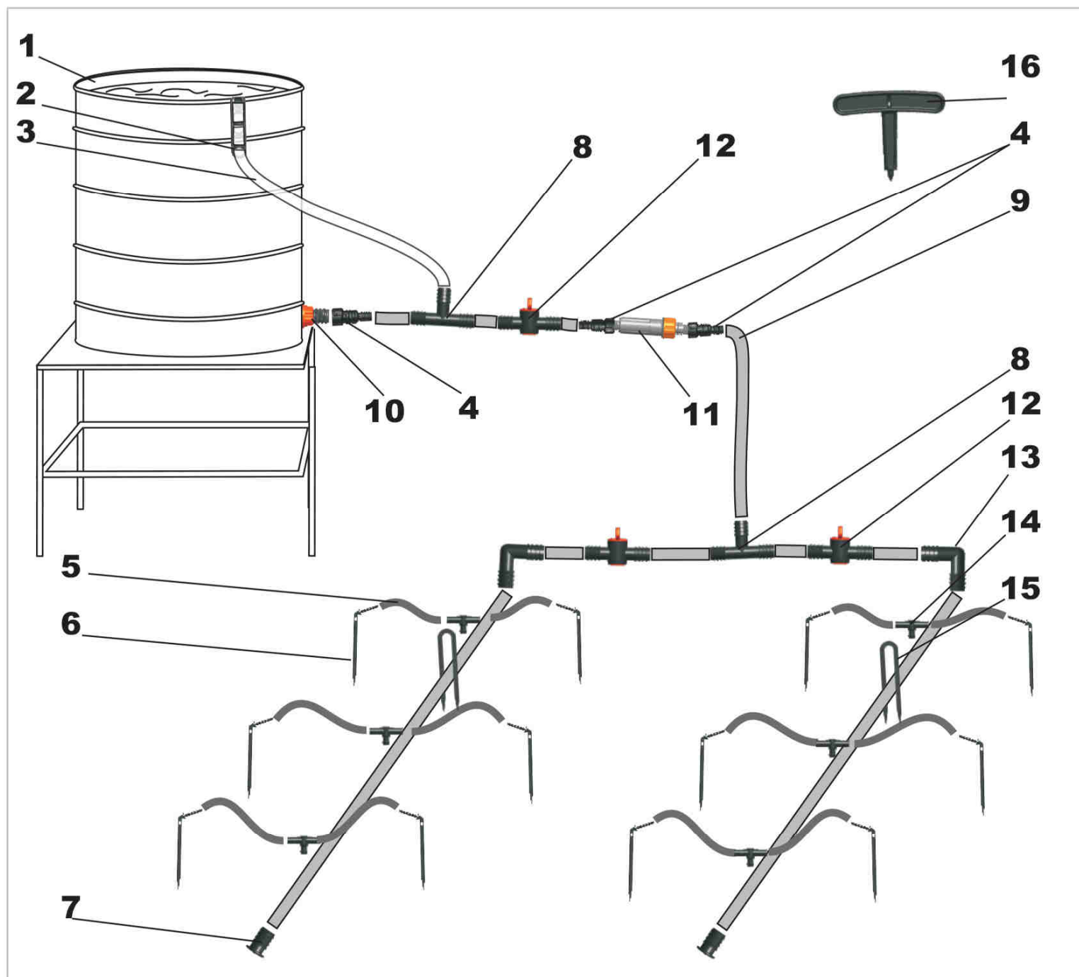
Рис. 1 Принципиальная схема сборки системы для капельного полива
